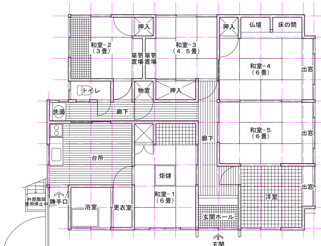
2 階平面図
