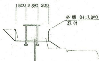
②-② 断面図
