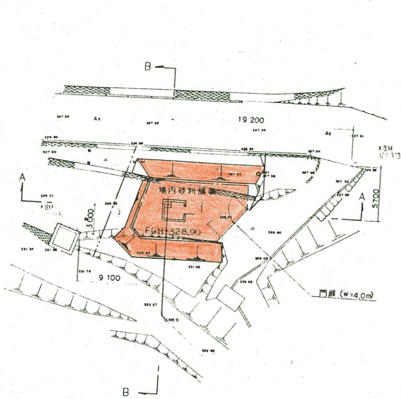
2号取水井平面図
