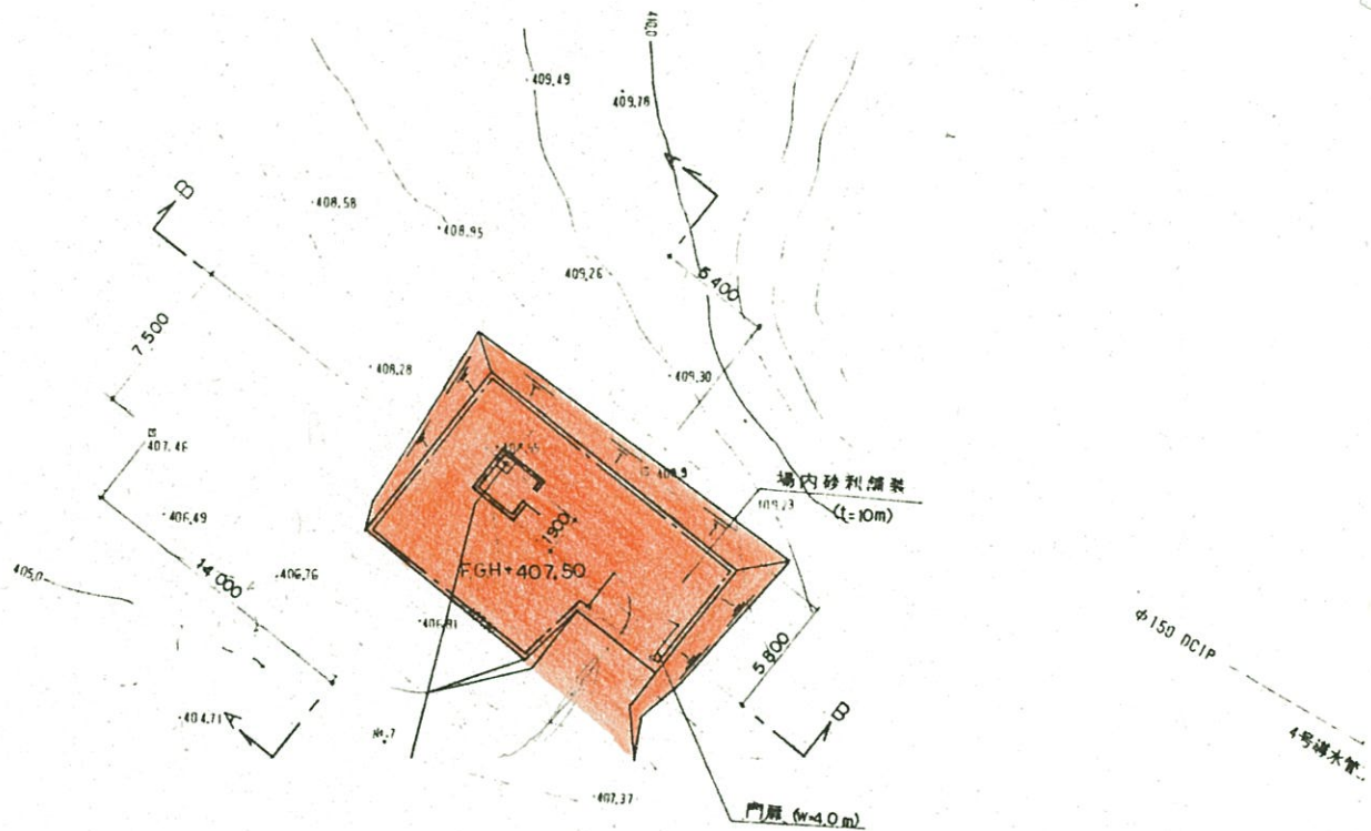
4号取水井平面图
