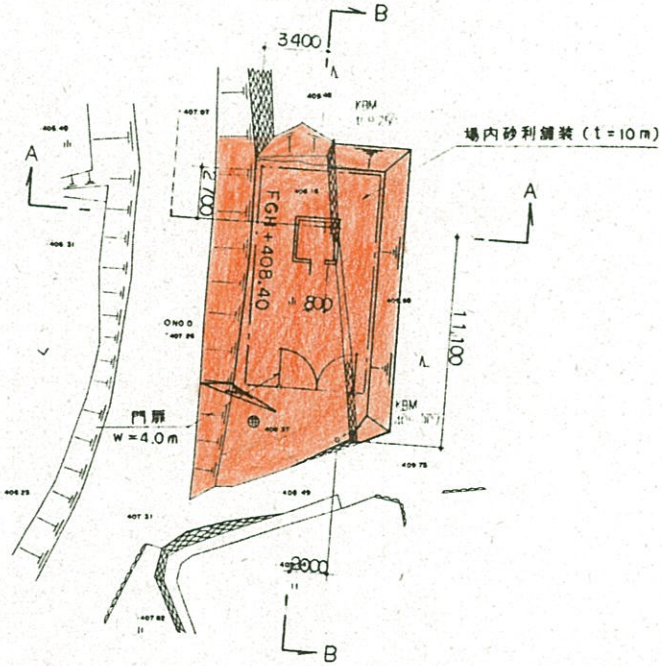
3号取水井平面図
