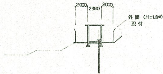
A-A 断面図
