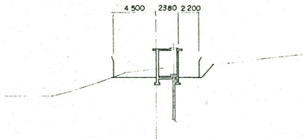
①-① 断面图
